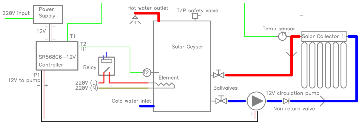
Fig 2. Wiring diagram.
